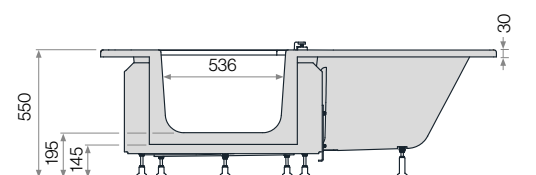
Kabino-wanna DUETT 160
